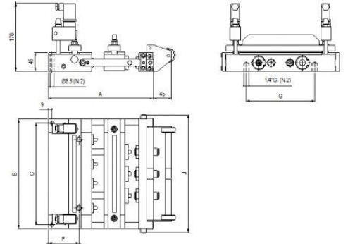
Dati dimensionali
