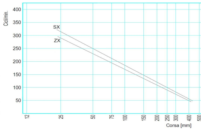
Diagramma cicli/minuto
